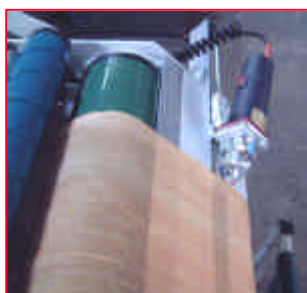
Pont support + outils de refente SW100 Alignement de lisière et détection fin de tissu
